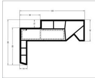
Blendrahmen 69-1
