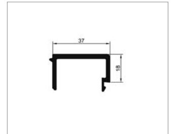
Halteprofil gestanzt/ungestanzt
