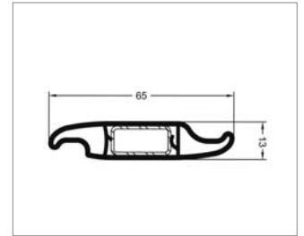
Kombi-Lamelle
