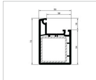
Flügel 72
