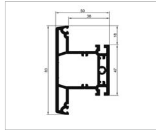
Sprosse 83
