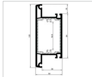
Sprosse 120
