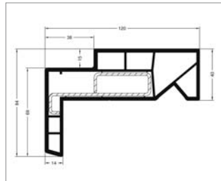
Blendrahmen 69-2
