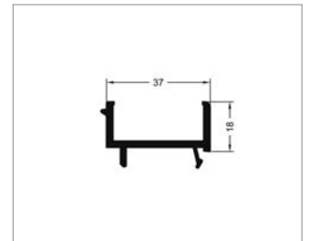
Halteprofil für bewegliche Lamelle
