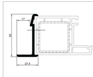
Stulpprofil
