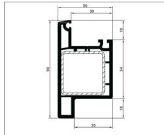
Flügel 90
