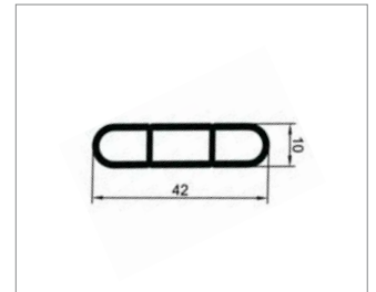
Lamelle 42
